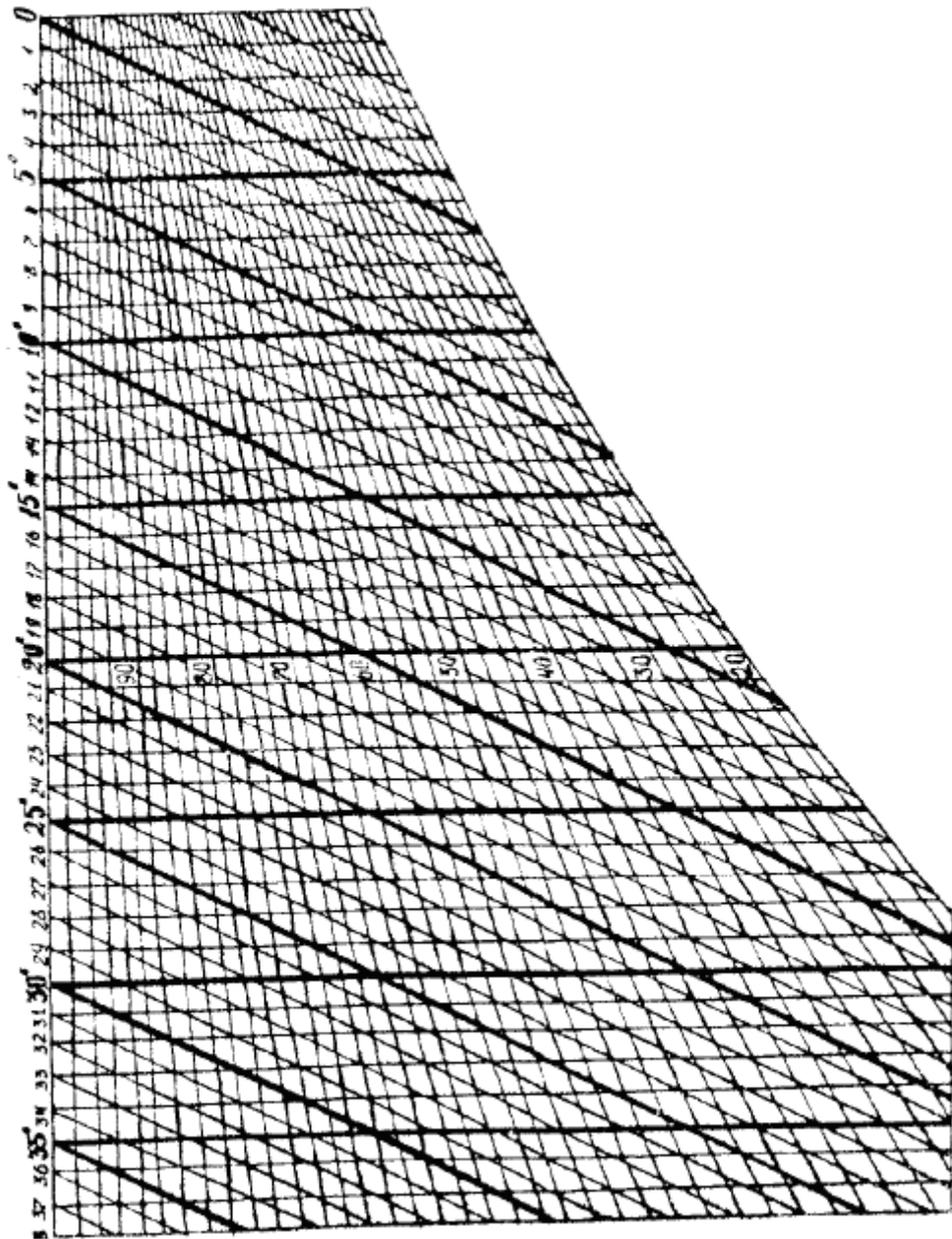
Рис. 3. Психрометрический график
