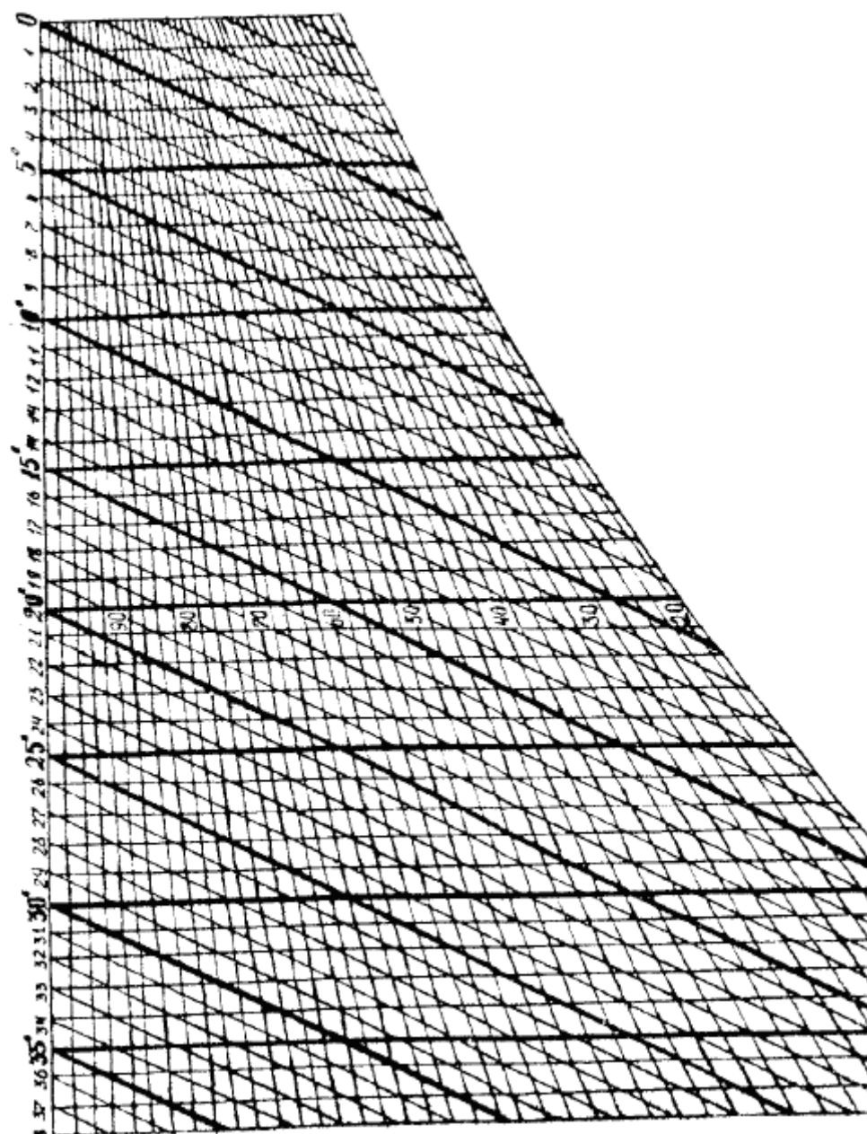
Рис. 3. Психрометрический график
