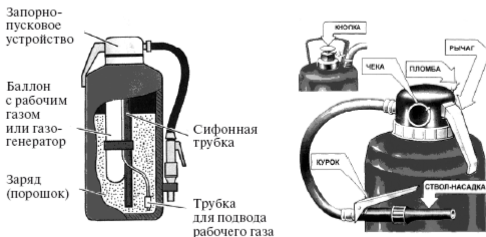
Рис. 11. Порошковый огнетушитель со встроенным газовым источником давления ОП-5
