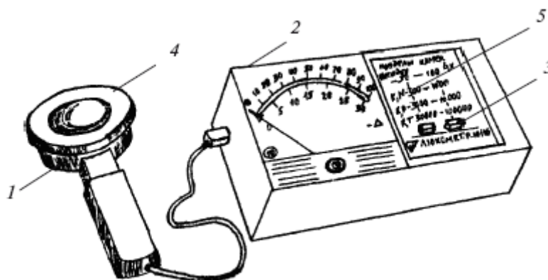
Рис. 8. Объективный люксметр
