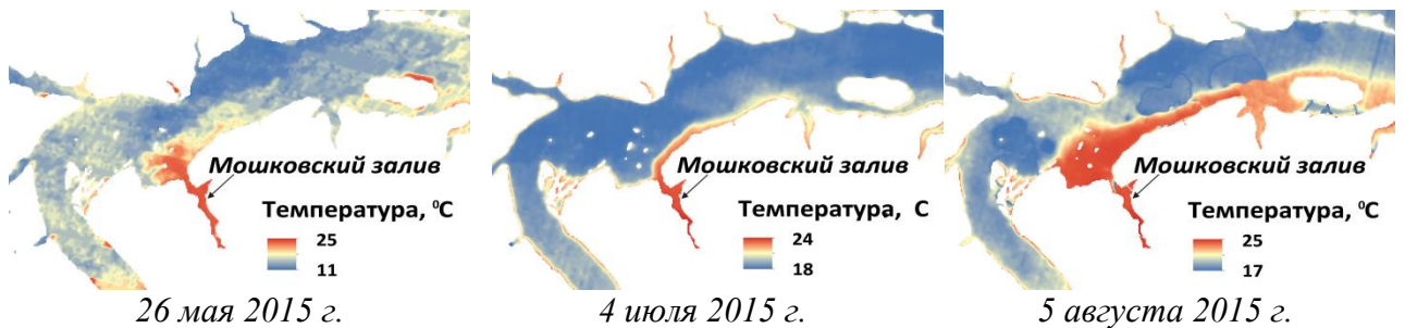
Рис. 12. Распределение температуры поверхностных вод в Мошковском заливе по данным сенсора TIRS спутника Landsat-8
