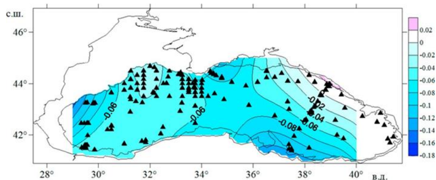
Рисунок 10 – Поле полуразностного композита величины рН для противоположных фаз ВАК в период с ноября по февраль за период 1957 по 1996 гг. (ВАК+ минус ВАК-)
