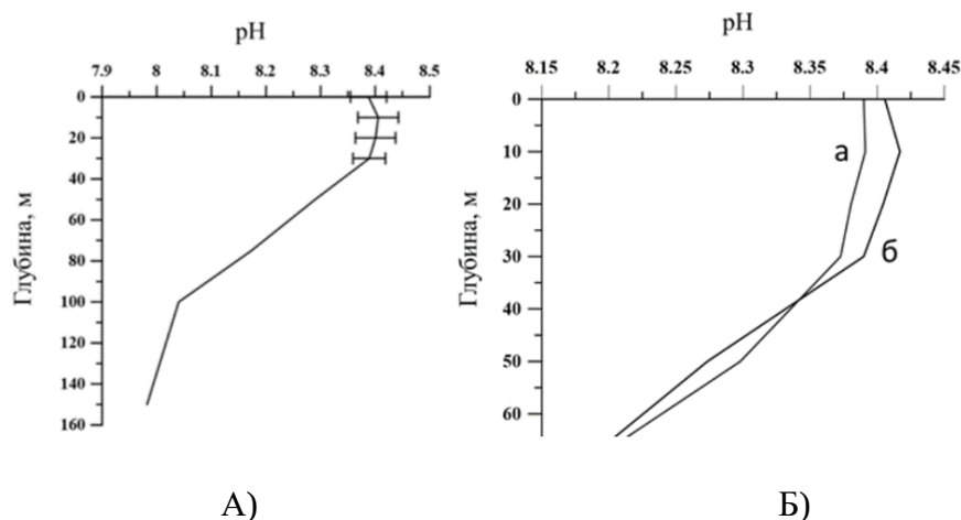
Рисунок 6 – Вертикальное климатическое распределение величины рН в слое 0–150 м с обозначенной величиной стандартного отклонения, обусловленного сезонной изменчивостью рН в верхнем 30-метровом слое (А) и усредненные профили величины рН в глубоководной части Черного моря (Б): а) январь – март; б) сентябрь – ноябрь
