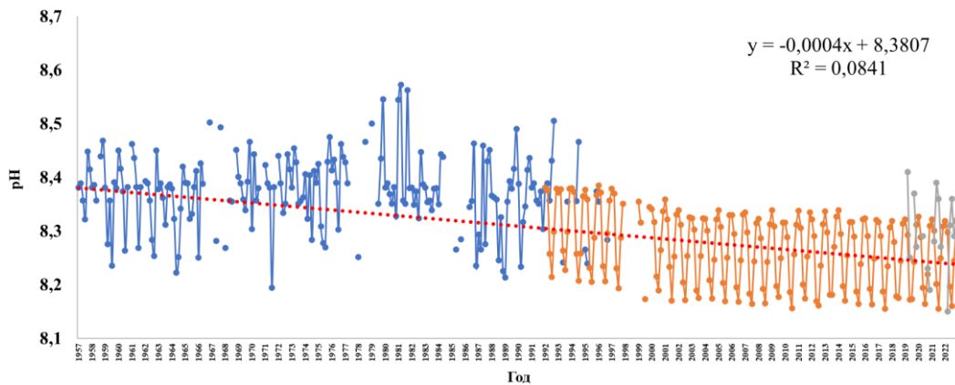
Рисунок 11 – График временного хода pH и уравнение линейного тренда, где x – шаг (период времени – 2 месяца) за 1957–2022 гг. Линейный тренд значим на уровне значимости 95%. Синий график – данные наблюдений в период 1957–1996 гг, оранжевый график данные о pH из ре-анализа CMEMS BS-Biogeochemistry, серый график – современные данные экспедиционных исследований 2019–2022 гг.
