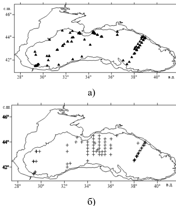
Рисунок 1 – Пространственное распределение станций, на которых измерялась величина рН на поверхности моря в августе 1966 г. (а) и декабре 1988 г. (б)
