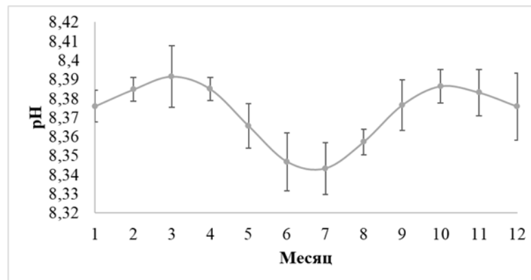
Рисунок 5 – Сезонный ход величины pH поверхностного слоя вод глубоководной части Чёрного моря. Вертикальные отрезки – среднеквадратическое отклонение среднемесячной величины pH
