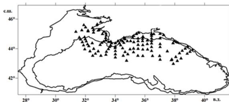
Рисунок 2 – Схема выполненных станций с фиксацией величины рН в ходе экспедиции НИС «Профессор Водяницкий» с 04 по 23 октября 2019 г.
